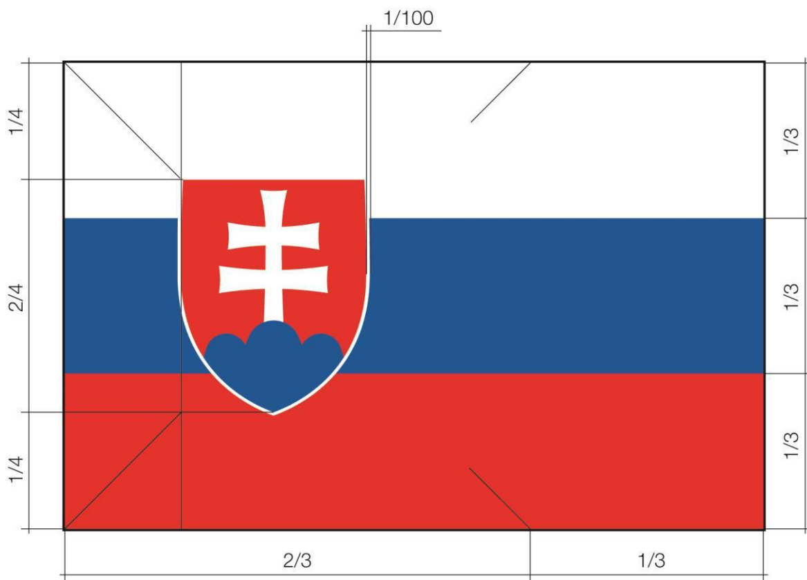
Štátna vlajka Slovenskej republiky – zostavovací nákres
